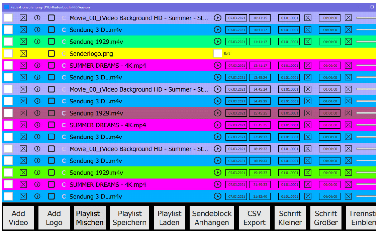
Abbildung: schnell durchschaubare, übersichtliche Planungsoberfläche
